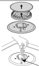
Инжектор
